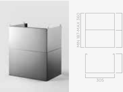
KIT CAMINO ACCIAIO INOX H185+H185 STAINLESS STEEL CHIMNEY KIT H185+H185
