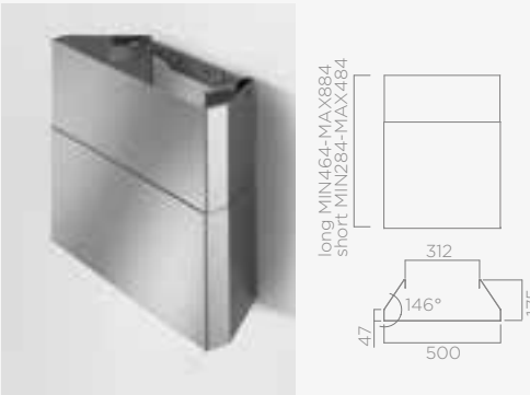
KIT CAMINO ACCIAIO INOX STAINLESS STEEL CHIMNEY KIT
