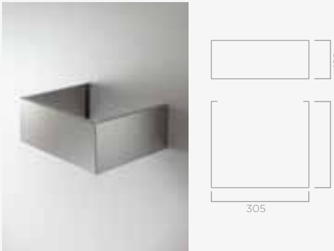
KIT CAMINO ACCIAIO INOX H12 STAINLESS STEEL CHIMNEY KIT H12
